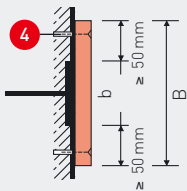
Profilflansch bündig mit Wandfläche
