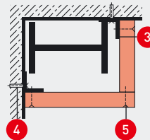
Zweiseitige Stützenbekleidung
