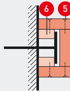
Stützenprofil teilweise vorstehend
