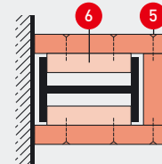
Dreiseitige Stützenbekleidung
